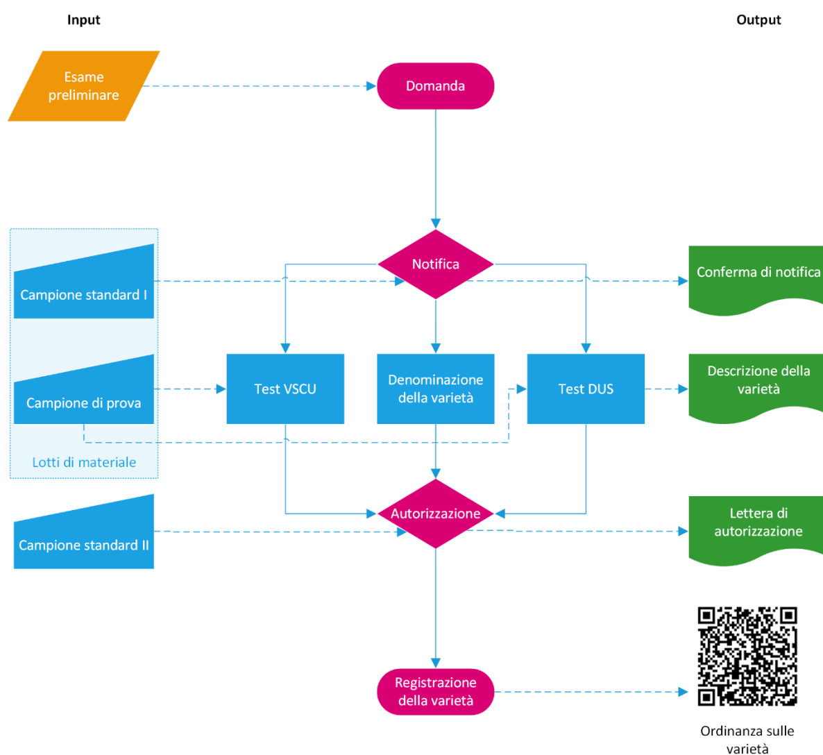
Figura 1 Iter ideale («Happy Path») dalla domanda alla registrazione
