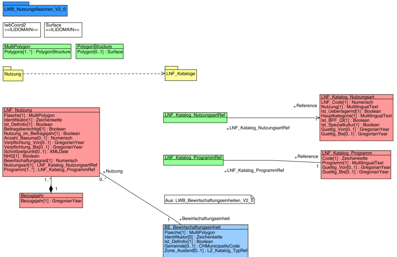
Figure 10 : Diagramme UML Surfaces d'utilisation
