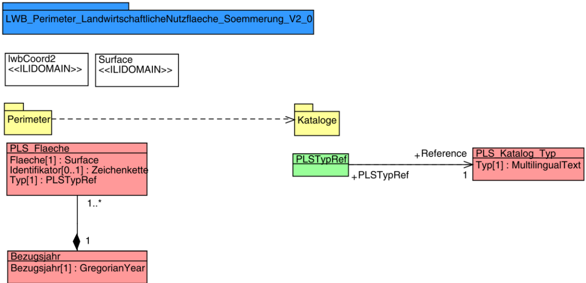
Figure 8 : Diagramme UML Périmètre Surface agricole utile et surfaces d'estivage
