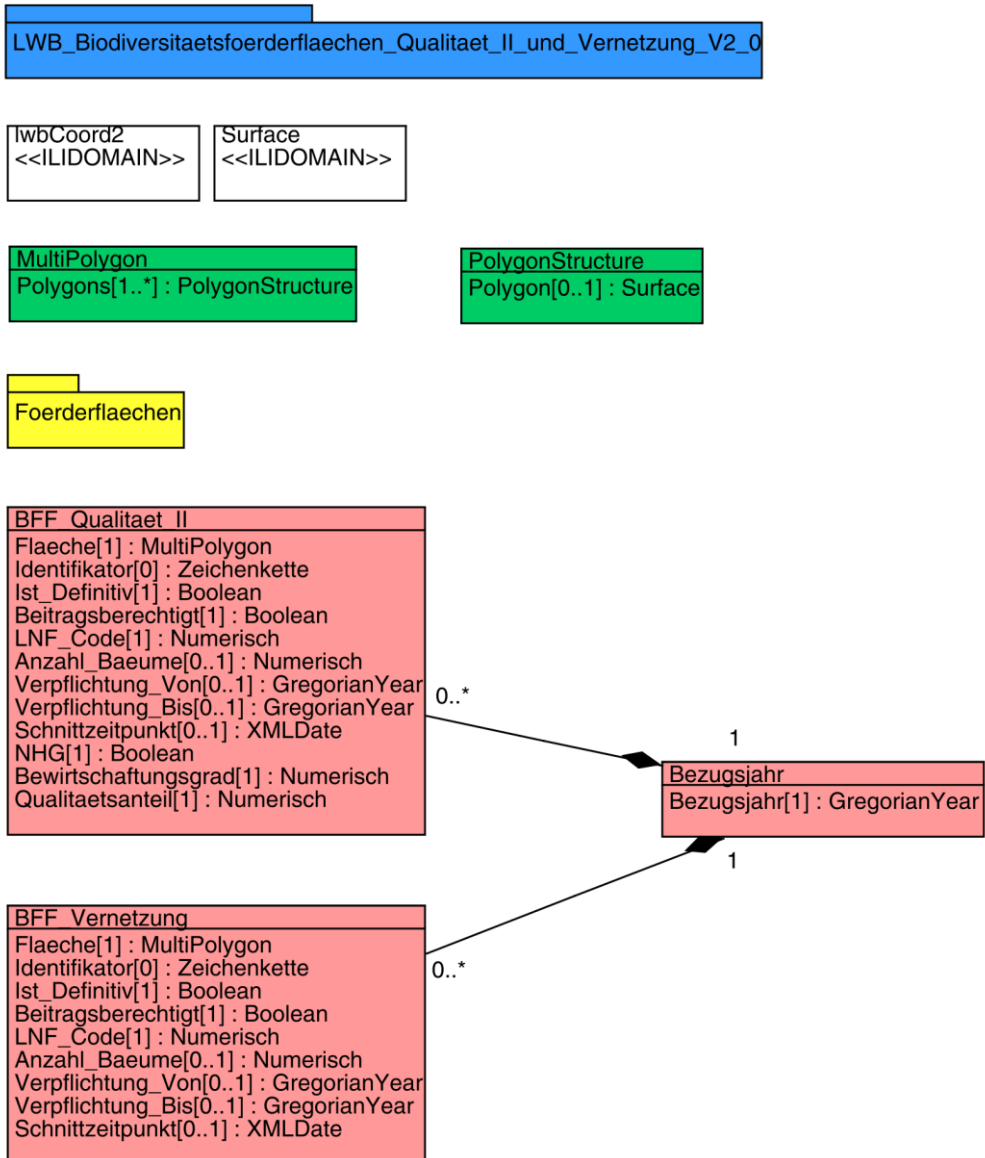
Figure 11 : Diagramme UML Surfaces de promotion de la biodiversité, niveau de qualité II et mises en réseau
